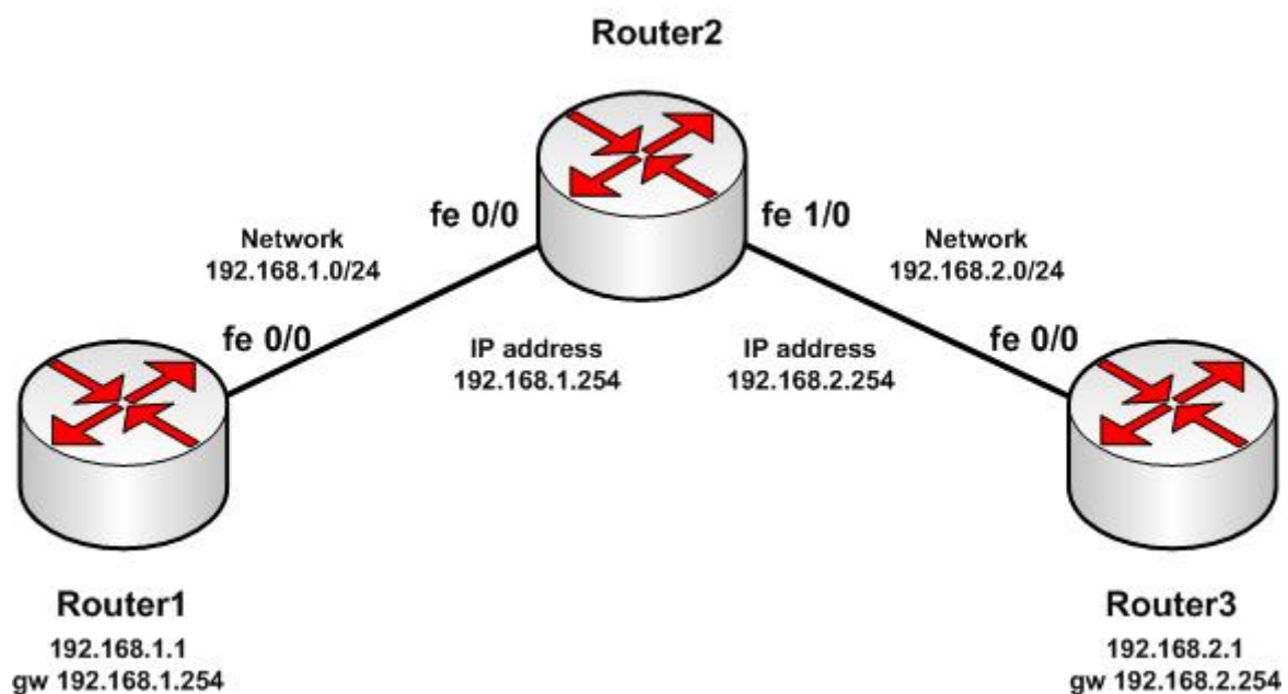
Propojení směrovačů v labu
